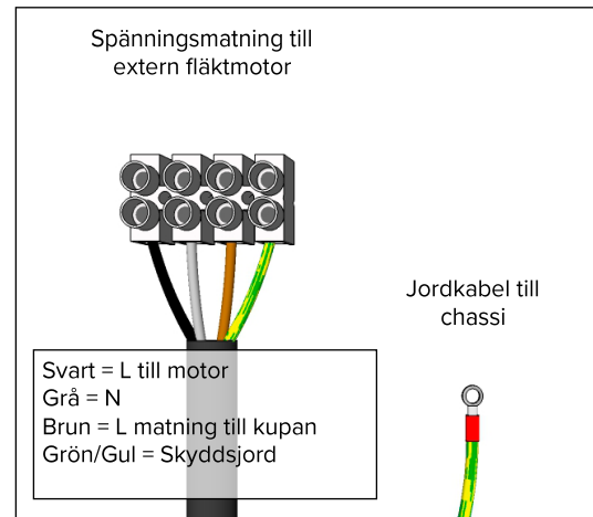
Fig 2. Koppling utan stickkontakt.
